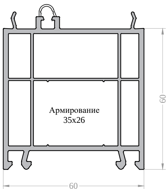
Профиль доборный 60/60 с уплотнением Арт. 10106060 *.25
