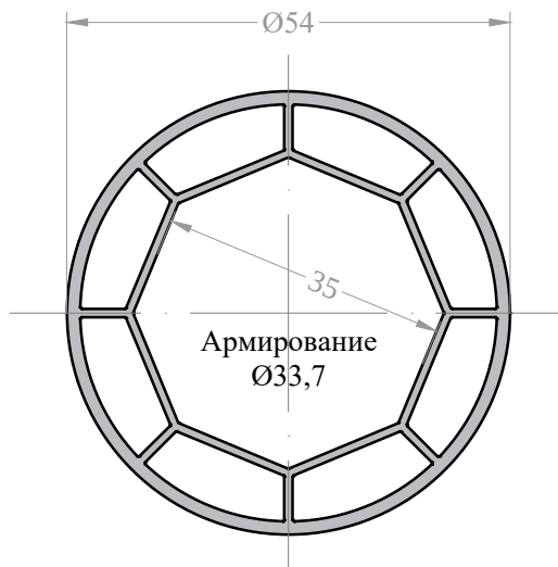
Труба эркерная Арт. 10105054 *
