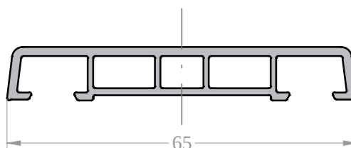
Наличник 65 Арт. 10106065 *
