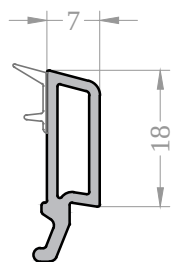
Штапик 7 AERO
