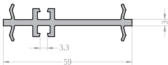
Профиль соединительный 3/60 Арт. 10105003
