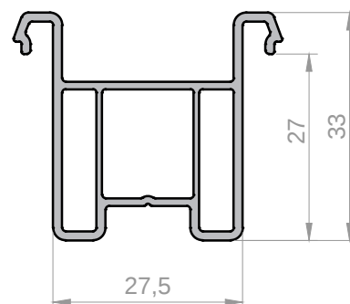
Профиль подставочный AERO Арт. 40006033
