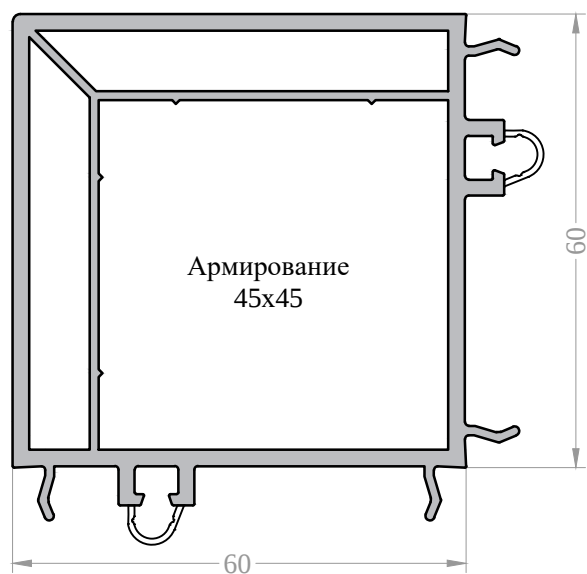
Профиль угловой 90/60 с уплотнением Арт. 10105060 *.255
