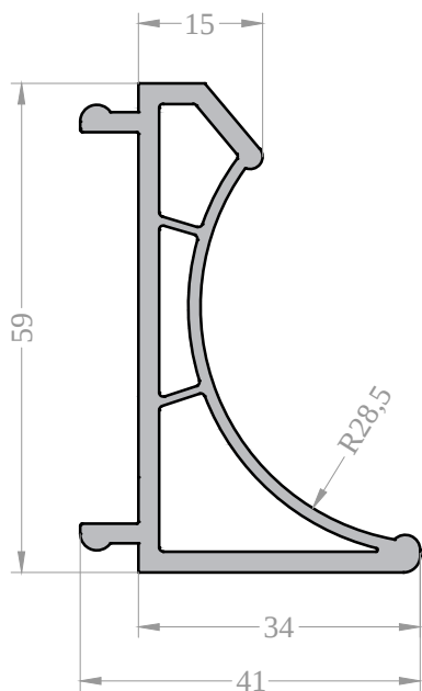
Профиль эркерный 60 Арт. 10105034 *
