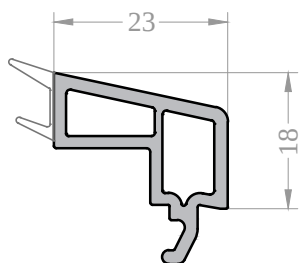
Штапик 23
