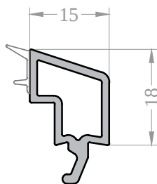
Штапик 15 AERO
