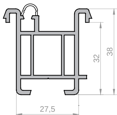
Профиль подставочный 30 с уплотнением Арт. 40106030.25 Арт. 40106030 - без уплотнителя
