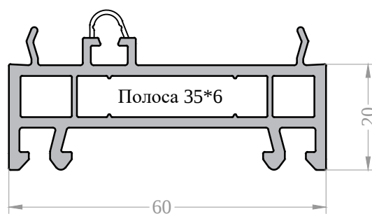
Профиль доборный 20/60 с уплотнением Арт. 10106020 *.25
