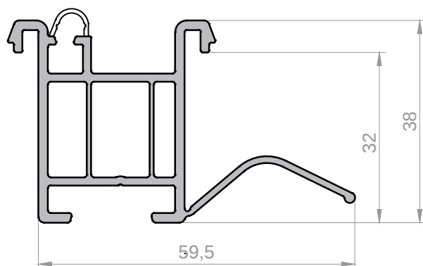
Профиль подставочный с опорной ножкой с уплотнением Арт. 40106060.25 Арт. 40106060 - без уплотнителя
