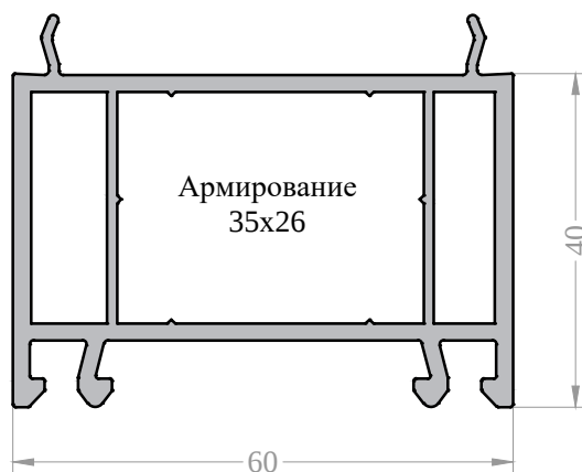
Профиль доборный 40/60 Арт. 10106040 *.25
