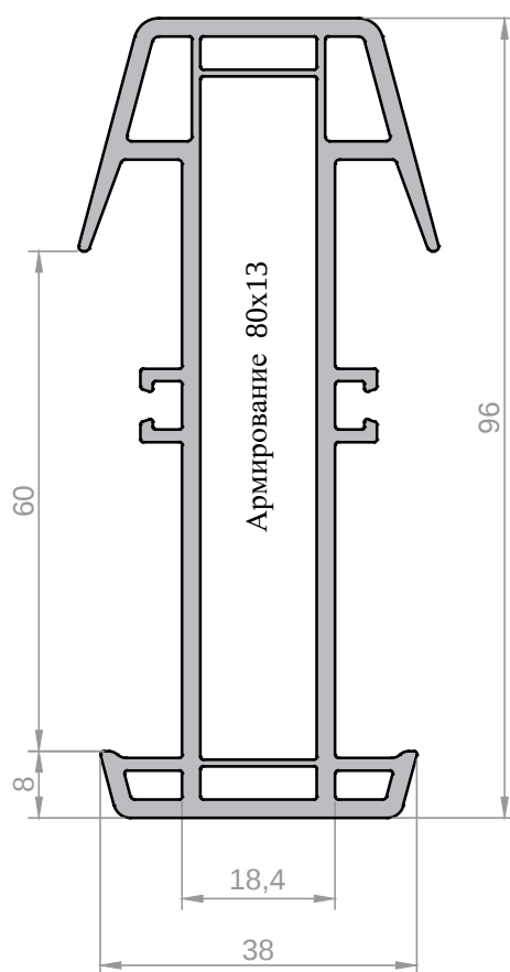
Профиль соединительный 38/60 Арт. 10105038 *
