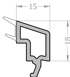
Штапик 15
