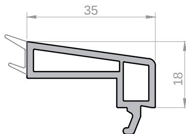
Штапик 35
