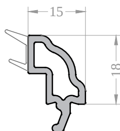
Штапик 15 фигурный
