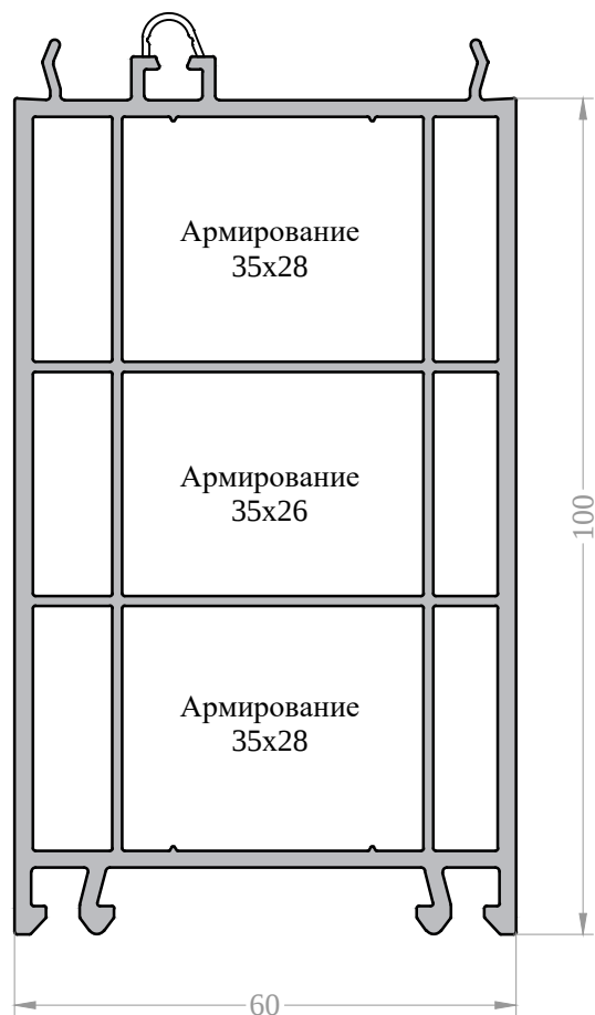
Профиль доборный 100/60 с уплотнением Арт. 10106100 *.25
