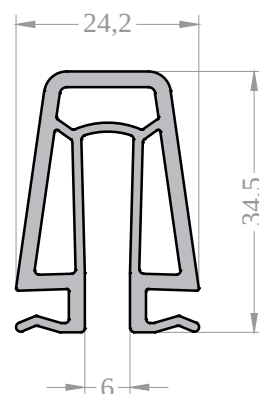
Профиль соединительный универсальный Арт. 10105024 *
