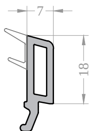
Штапик 7
