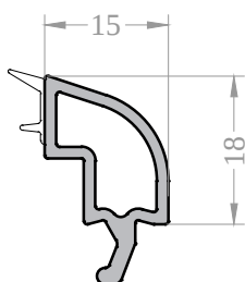
Штапик 15 круглый
